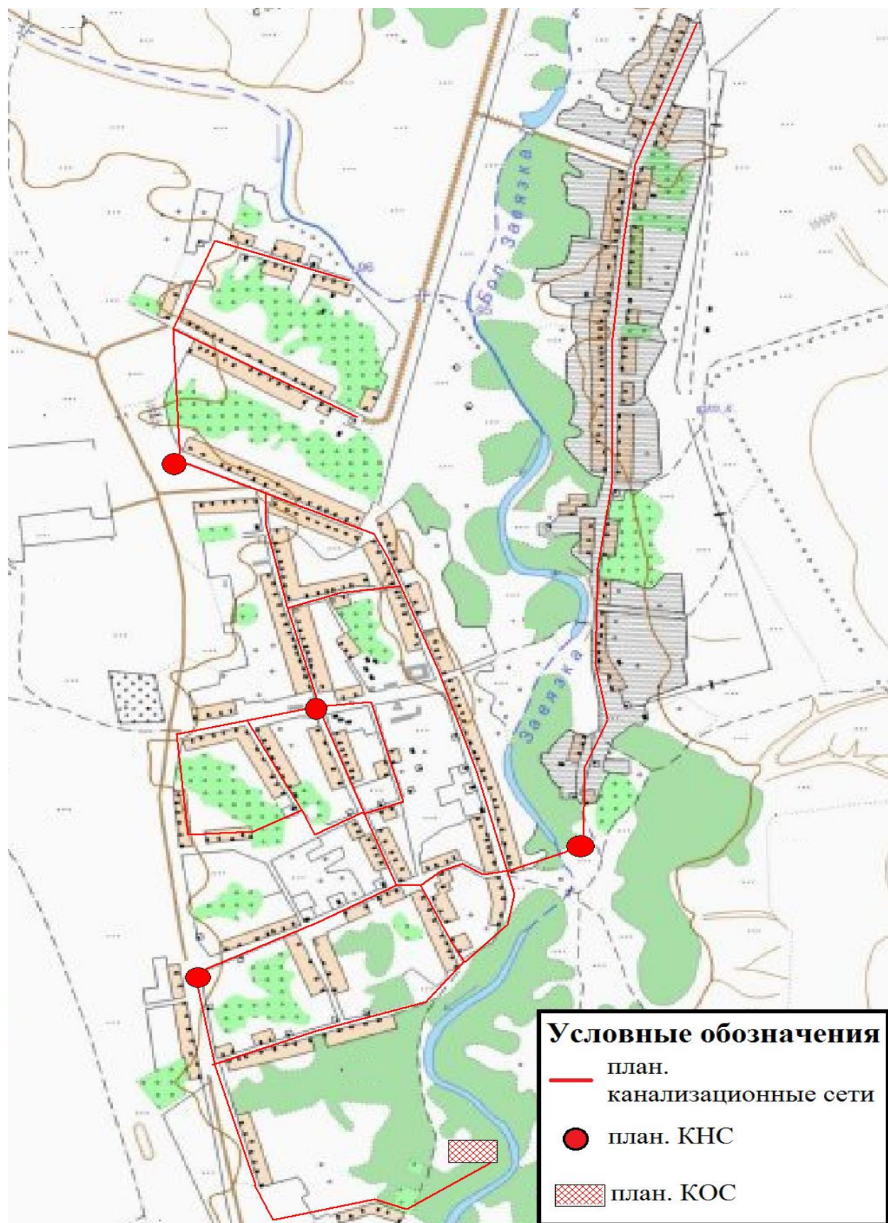
Рис. 3 Планируемая система водоотведения с. Завязка
